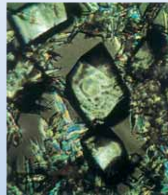
Kristali kalcijevega karbonata, obdelani s Polarjem, so srijeti in potujejo naprej skupaj z vodo brez nalaganja na cevi
